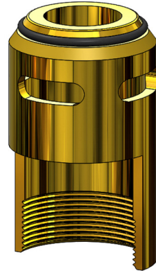
Standard Barrel 27218-07 1.99" High, 1.175" OD OEM: 27218-07
