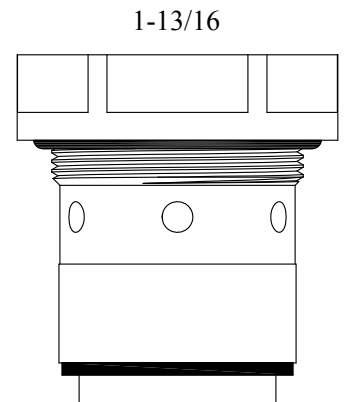
647640 SYMMONS C-3*
