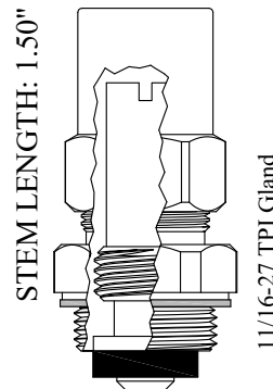
400321
