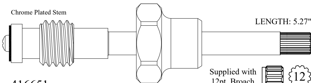
416651 216651 Stem Only
