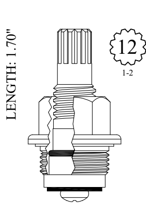
LF453401
