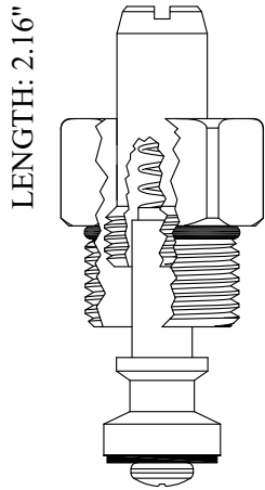
LF400571 OEM # 2755-005-002 LF200571 Stem Only OEM # 2755-005-002
