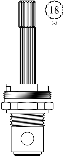
Cap Nut # 702510 available
