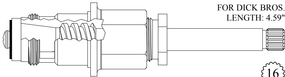
430611 230611 Stem Only GASKET: 895350
