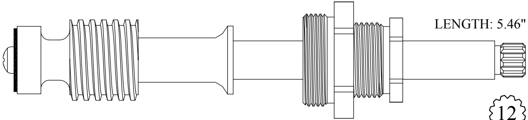
420751 220751 Stem Only GASKET: 895550
