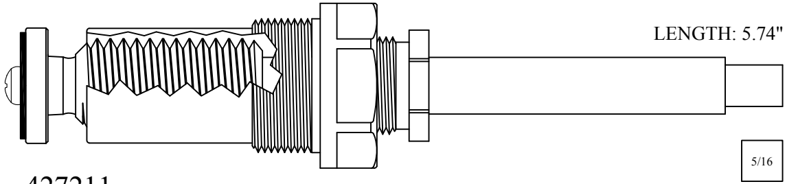
427211 227211 Stem Only GASKET: 895540
