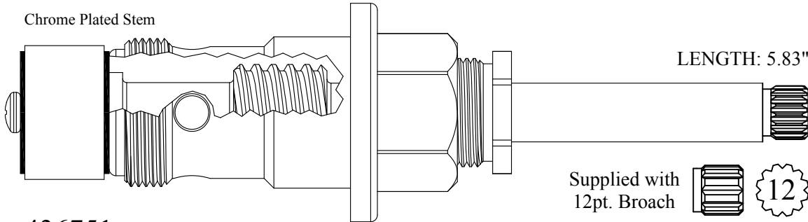
436751 236751 Stem Only GASKET: 895450
