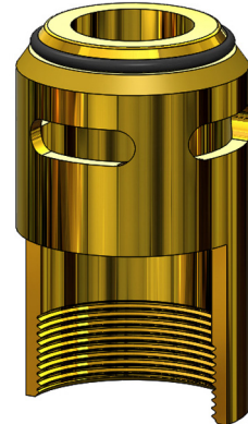
Standard Barrel 27218-07 1.99" High, 1.175" OD OEM: 27218-07
