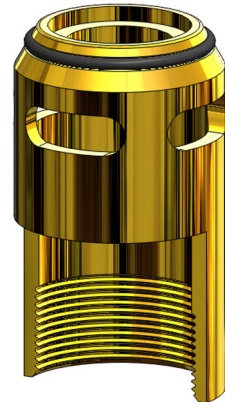
Standard Barrel 27221-07 1.98" High, 1.155" OD OEM: 27221-07
