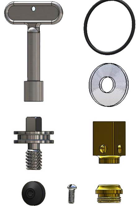
Z1300 & Z1310 Repair Kit 149650
